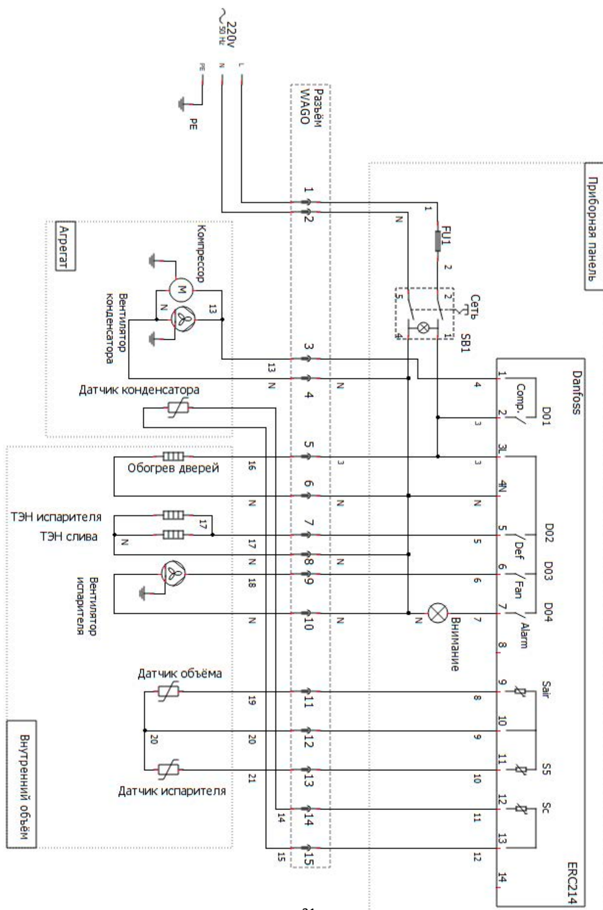
Рисунок 2. Схема электрическая для НХС
